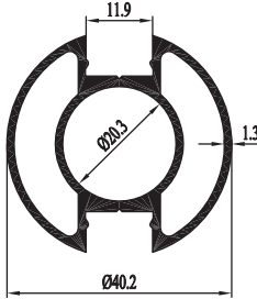
62 2123 00 0.061 kg/m
