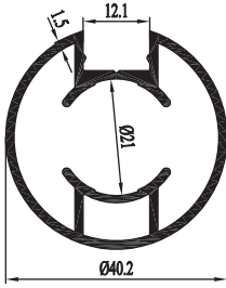
62 5321 00 0.770 kg/m
