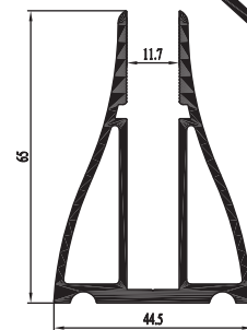
62 5400 00 1.898 kg/m
