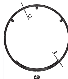
62 4945 00 0.602 kg/m
