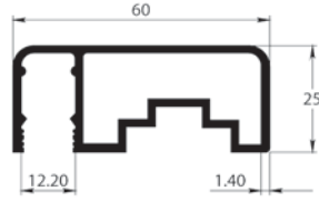
K-8037 0.800 kg/m
